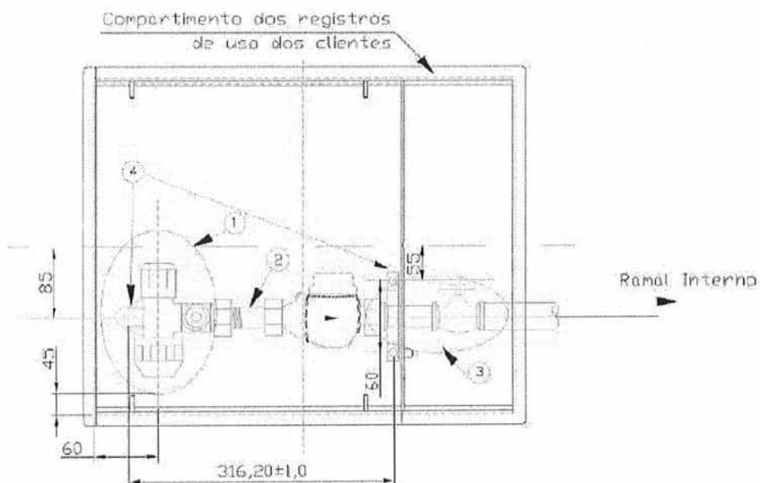
Figura 1 – Desenho esquemático de um dispositivo de medição
