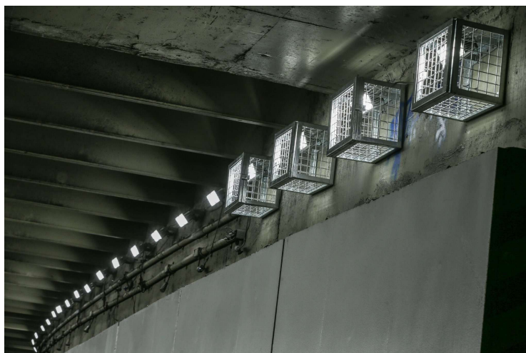
Caixas gradeadas usadas no Rio de Janeiro para conter vandalismo.
